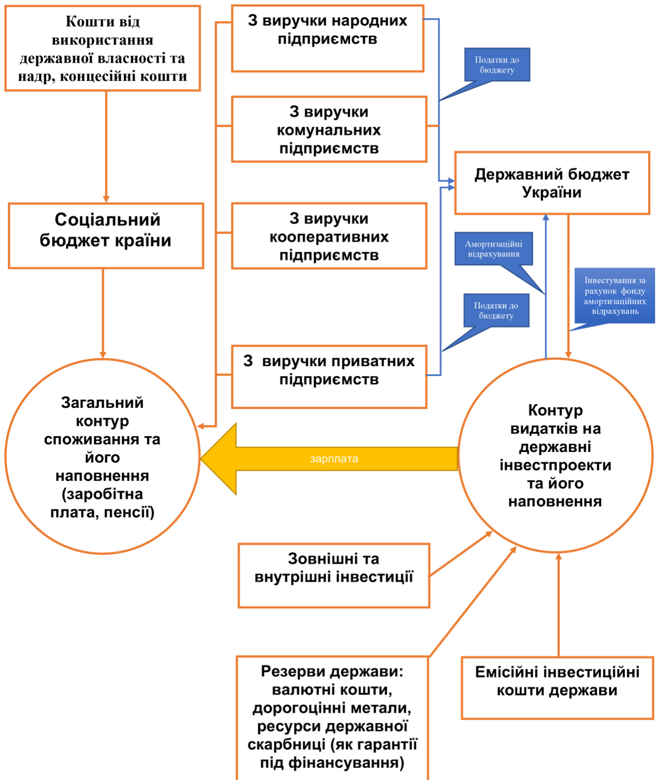
СХЕМА 1. Грошовий обіг країни
